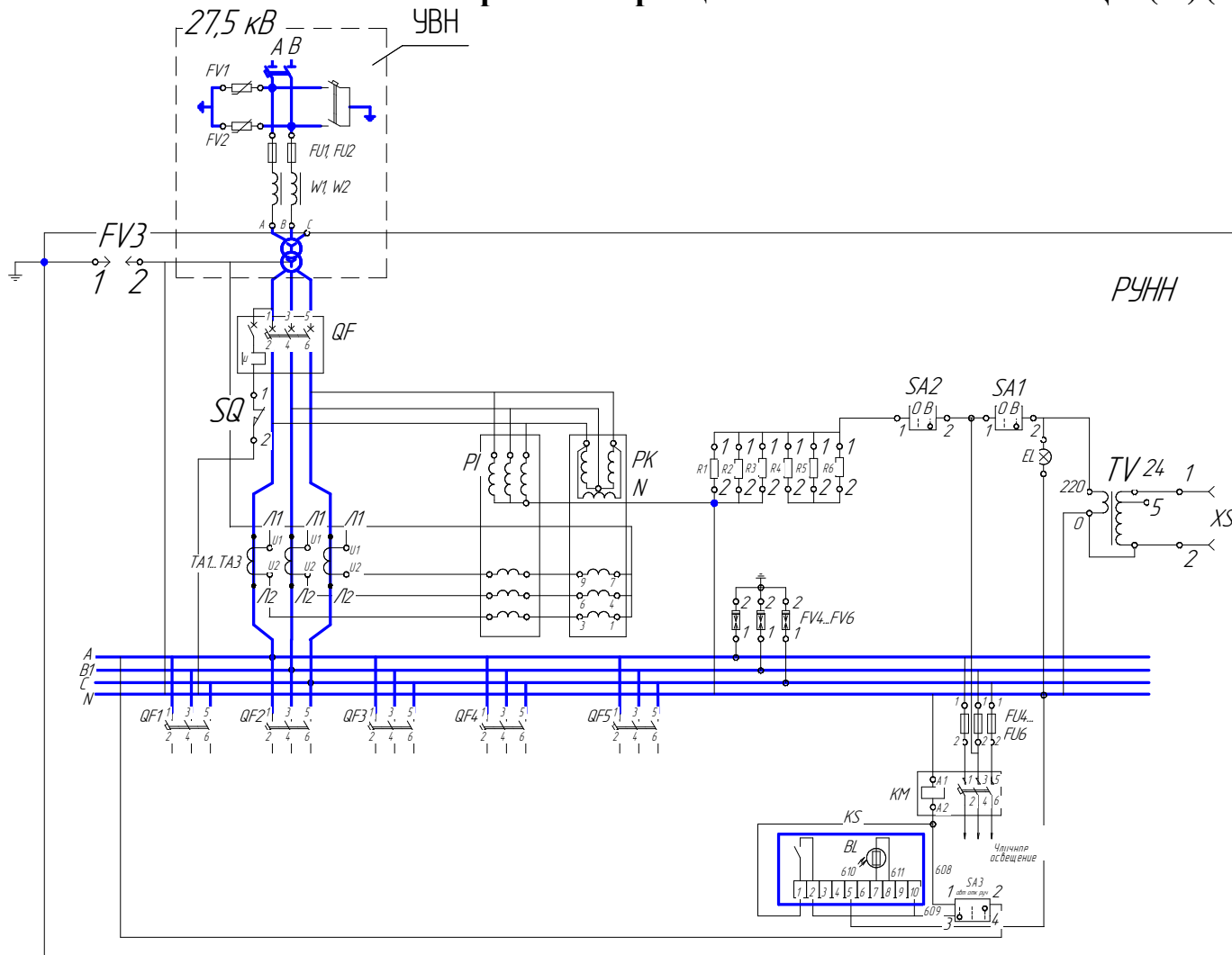
Рисунок А.1 – Схема электрическая принципиальная КТП СЭЩ Ж(М)-□/27,5/0,4-2006- 1
