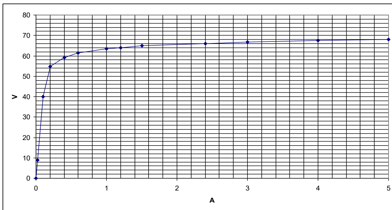
ВАХ вторичной обмотки для защиты с КТ 10Р, номинальной нагрузкой 15 ВА и K_{\text{ном}}=10 трансформаторов с первичными токами 3000 А. Сопротивление обмотки постоянному току – 0,46 Ом
