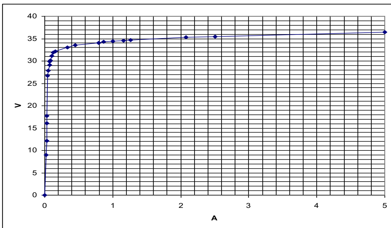
ВАХ вторичной обмотки для защиты с КТ 10Р, номинальной нагрузкой 15 ВА и K_{ном}=10 трансформаторов с первичными токами 2000 А. Сопротивление обмотки постоянному току – 0,35 Ом
