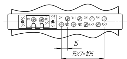
Рис. 2 Остальное см. рис. 1 (Исполнение с пятью вторичными обмотками) А
