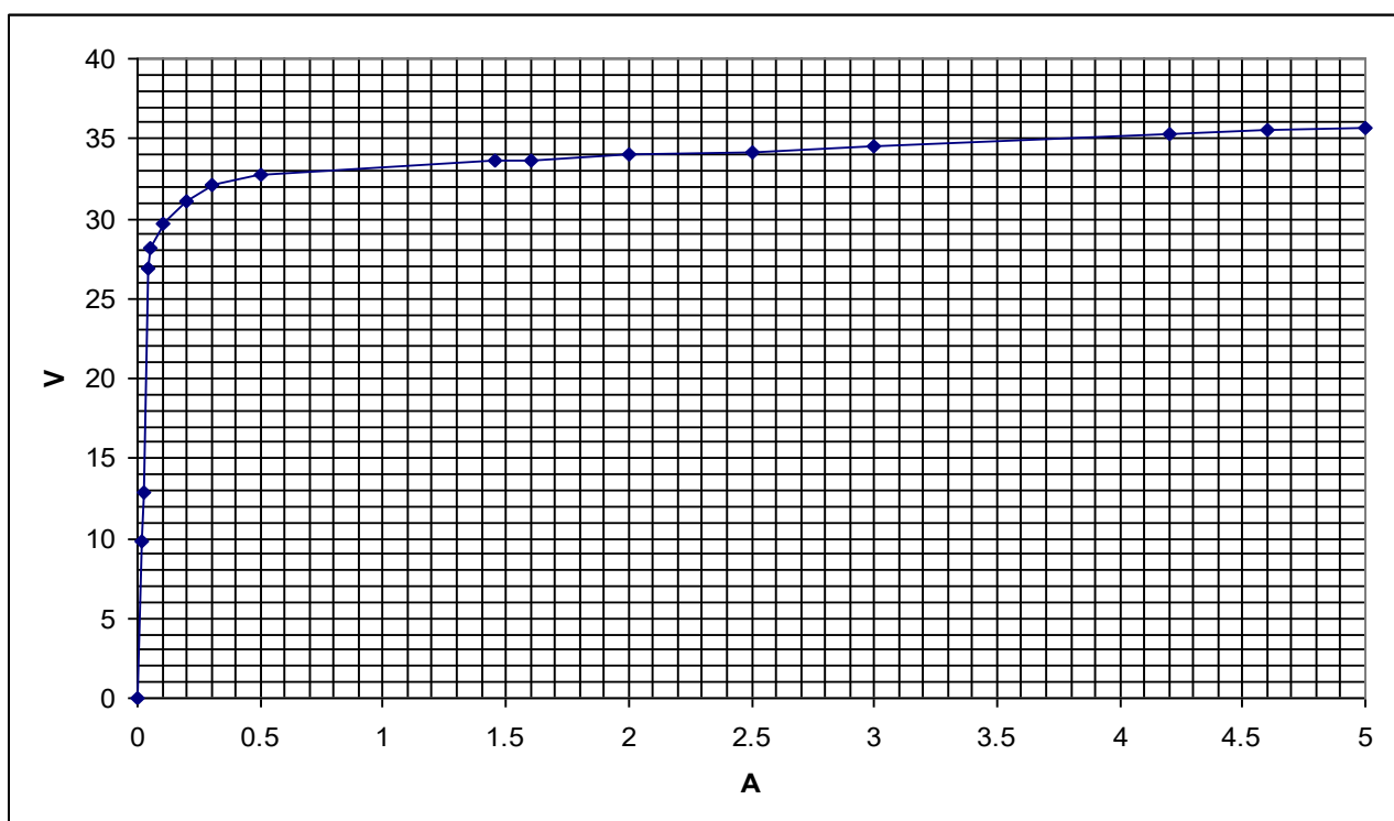
ВАХ вторичной обмотки для измерения с КТ 0,5; 0,5S; 0,2, 0,2S, номинальной нагрузкой 10ВА и K_{бном}=10 трансформаторов с первичными токами 3000 А. Сопротивление обмотки постоянному току – 0,43 Ом.
