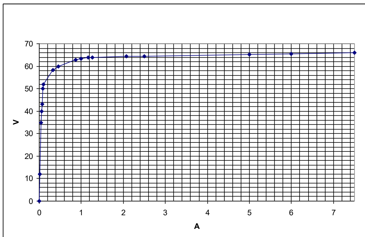
ВАХ вторичной обмотки для измерения с КТ 0,5; 0,5S; 0,2, 0,2S, номинальной нагрузкой 20ВА и K_{\text{Бном}}=15 трансформаторов с первичными токами 4000 А. Сопротивление обмотки постоянному току – 0,57 Ом.
